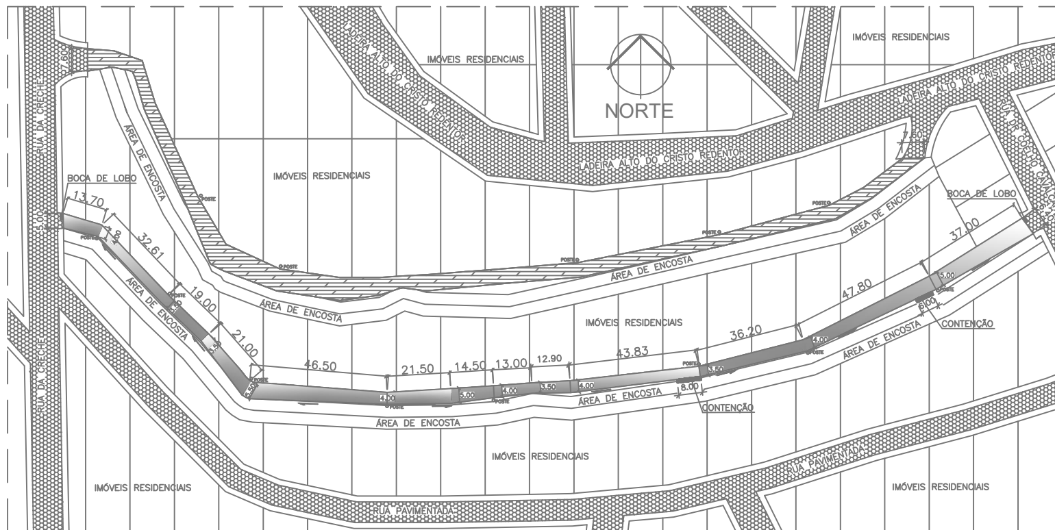
1 PLANTA DE LOCALIZAÇÃO DA RUA A SER PAVIMENTADA 1:1000
