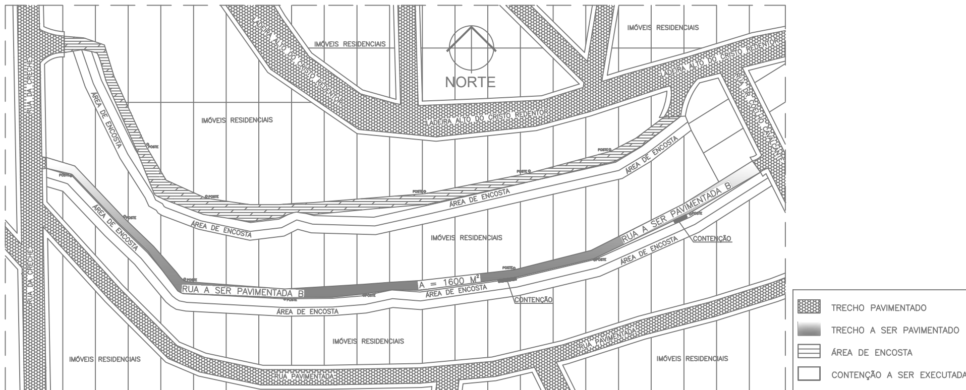
1 PLANTA DE LOCALIZAÇÃO DA RUA A SER PAVIMENTADA 1:1000
