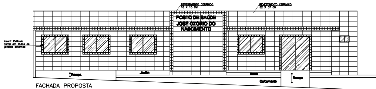
FACHADA PROPOSTA
