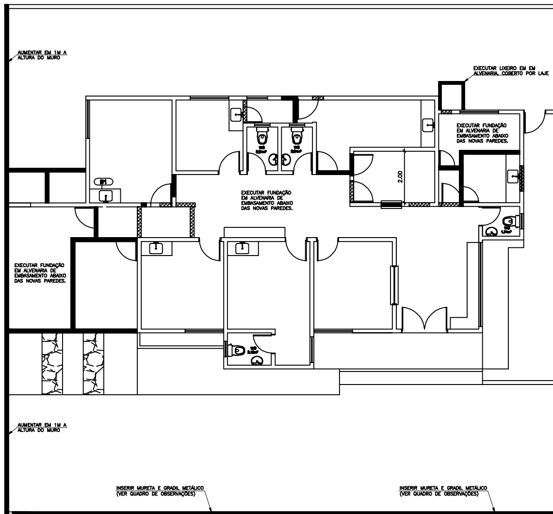
PLANTA BAIXA DEMOLIR-CONSTRUIR ESCALA _____ 1/75
