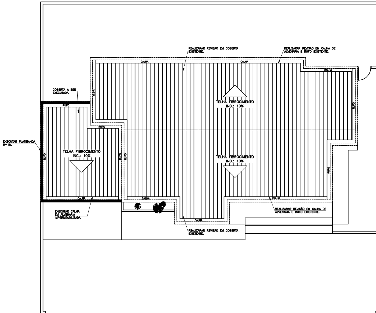
PLANTA DE COBERTA ESCALA _____ 1/75
