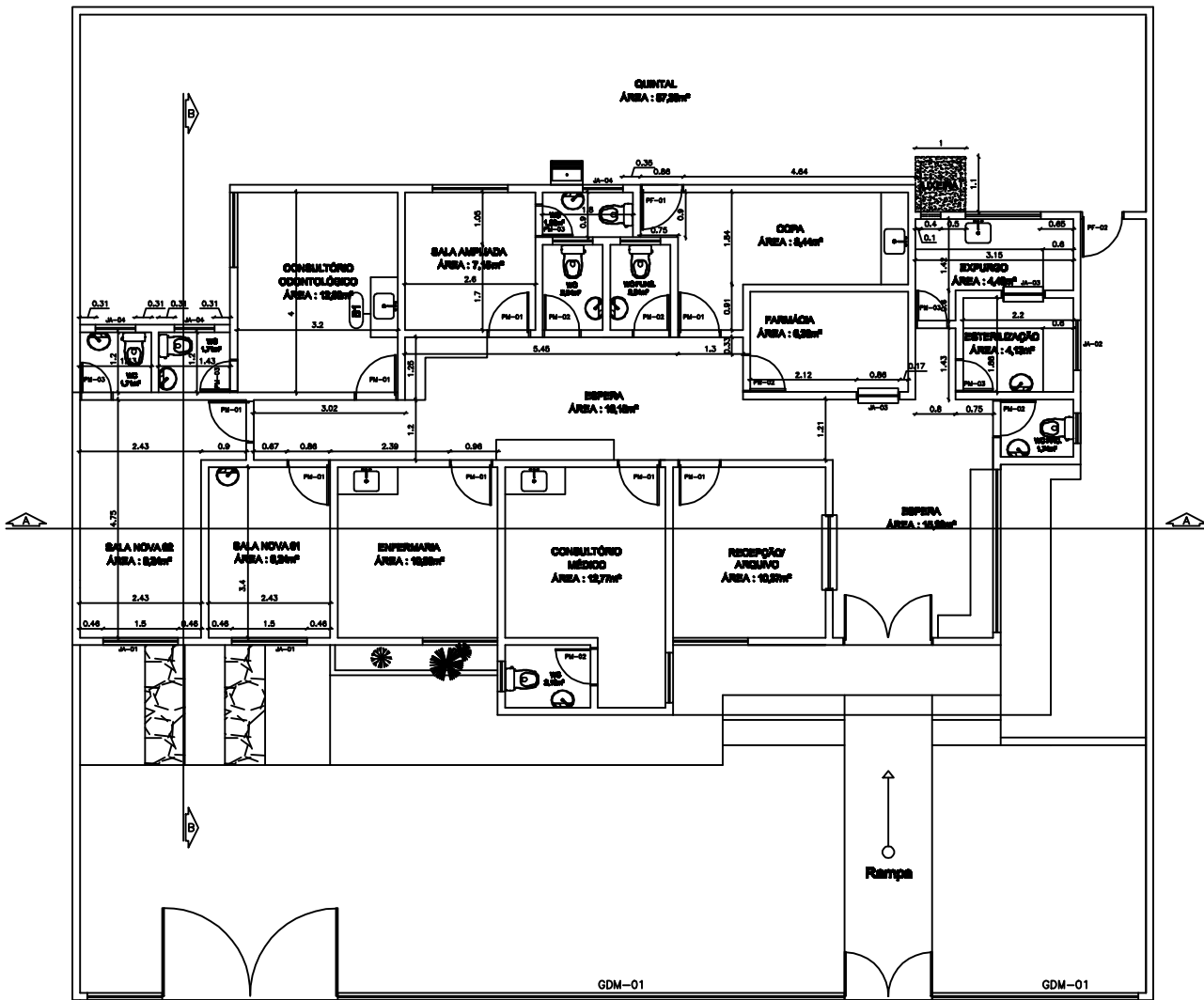
PLANTA BAIXA COTADA ESCALA _____ 1/75
