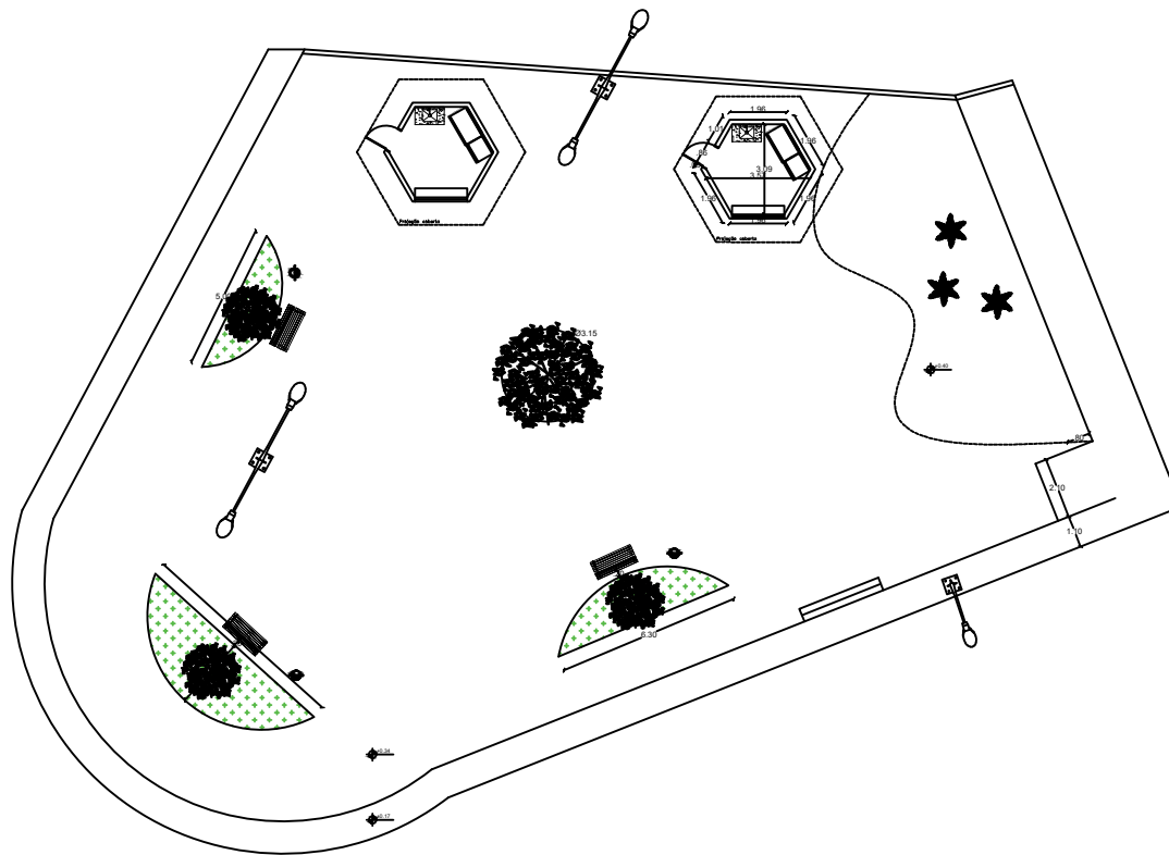
PLANTA BAIXA - ATUAL esc 1:50
