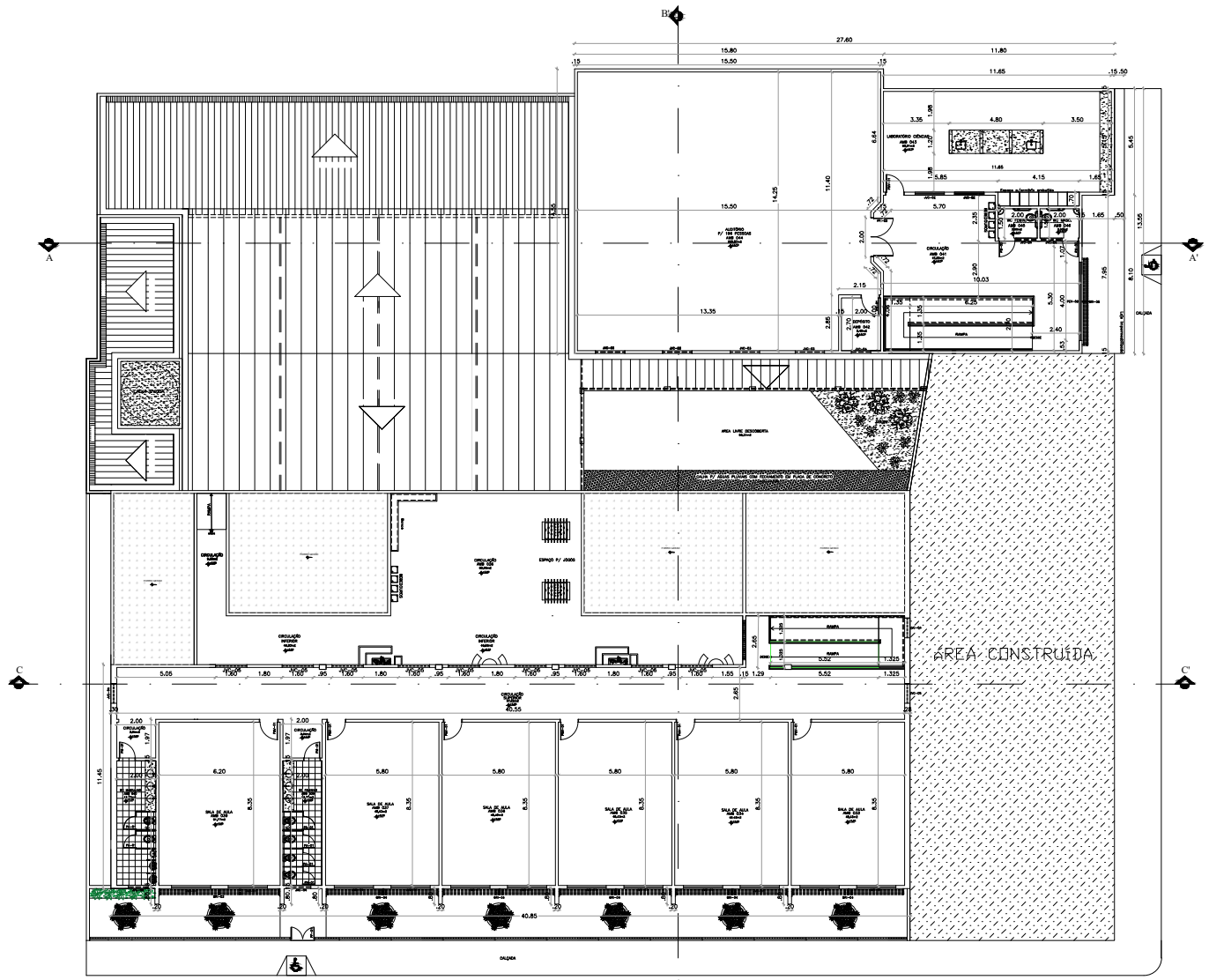
PLANTA-BAIXA REFORMA – PAVIMENTO SUPERIOR ESCALA 1/100
