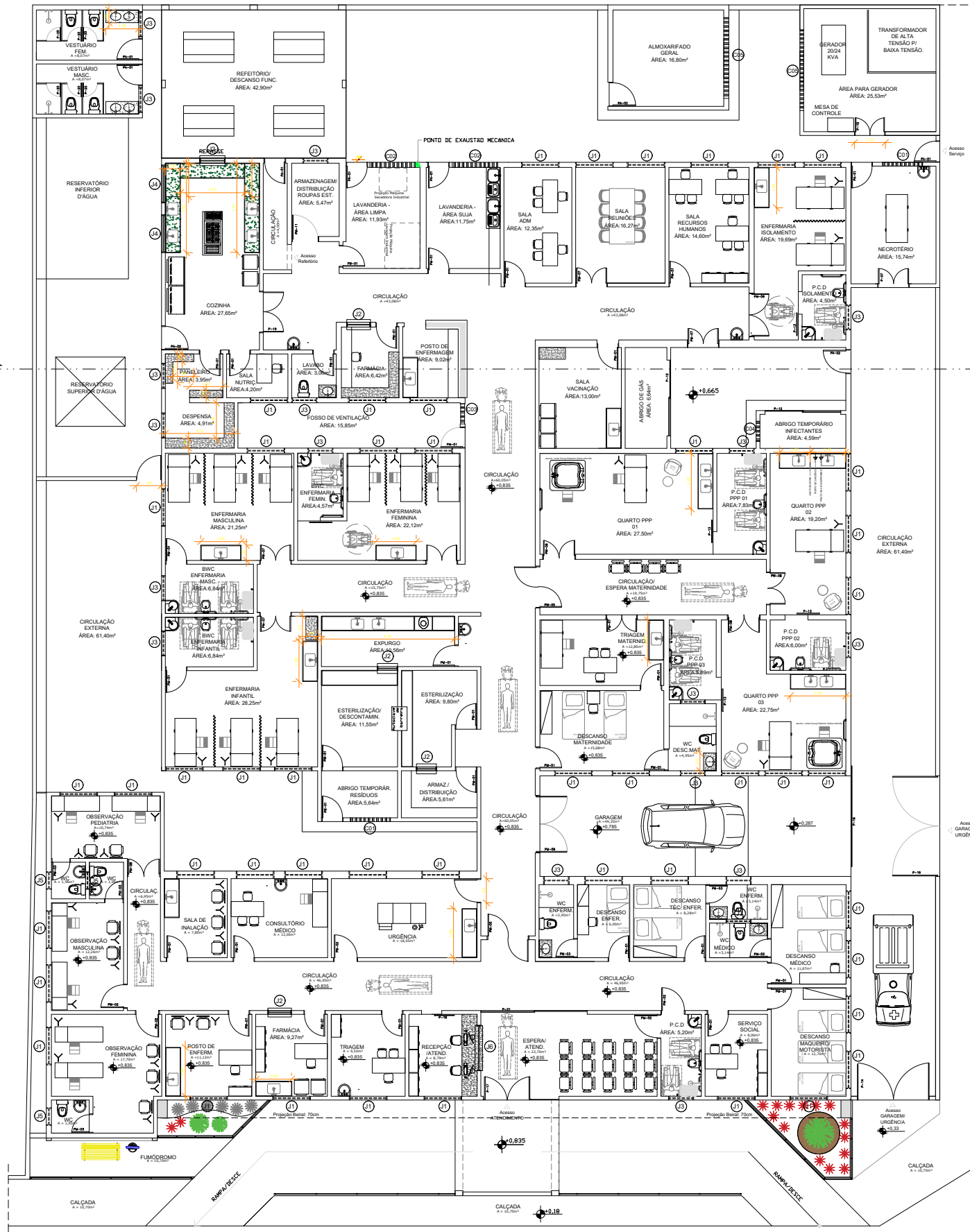
PLANTA DE LAYOUT - PROPOSTA REFORMA ESCALA 1/100
