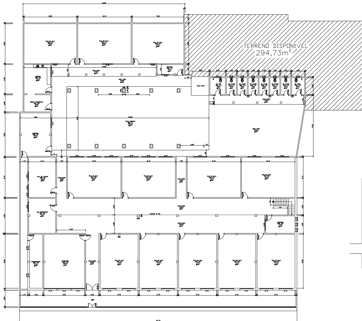
LEVANTAMENTO PLANTA ATUAL PAV. TÉRREO E TERRENO DISPONÍVEL ESCALA 1/100
