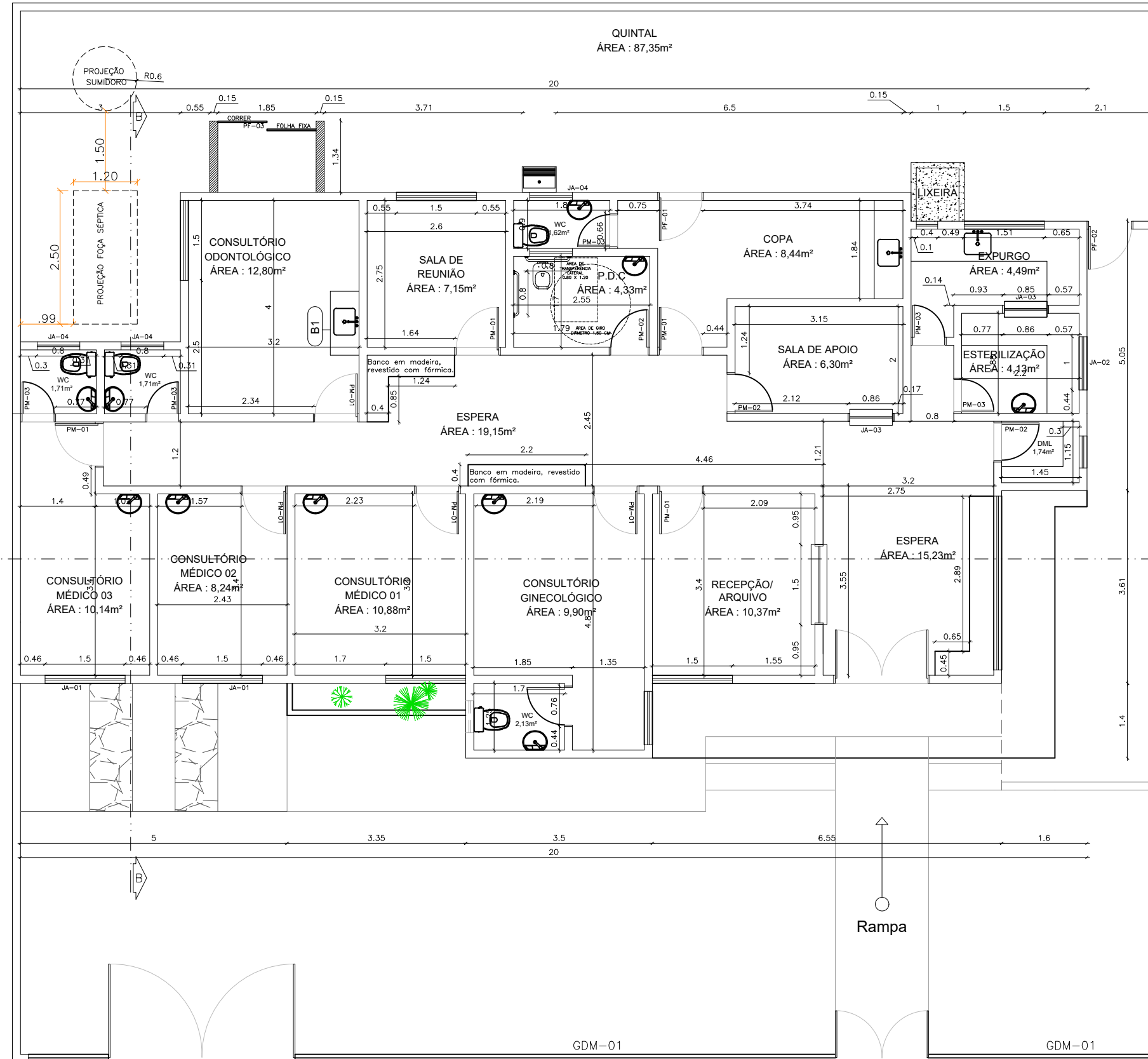
PLANTA BAIXA COTADA ESCALA _____ 1/75
