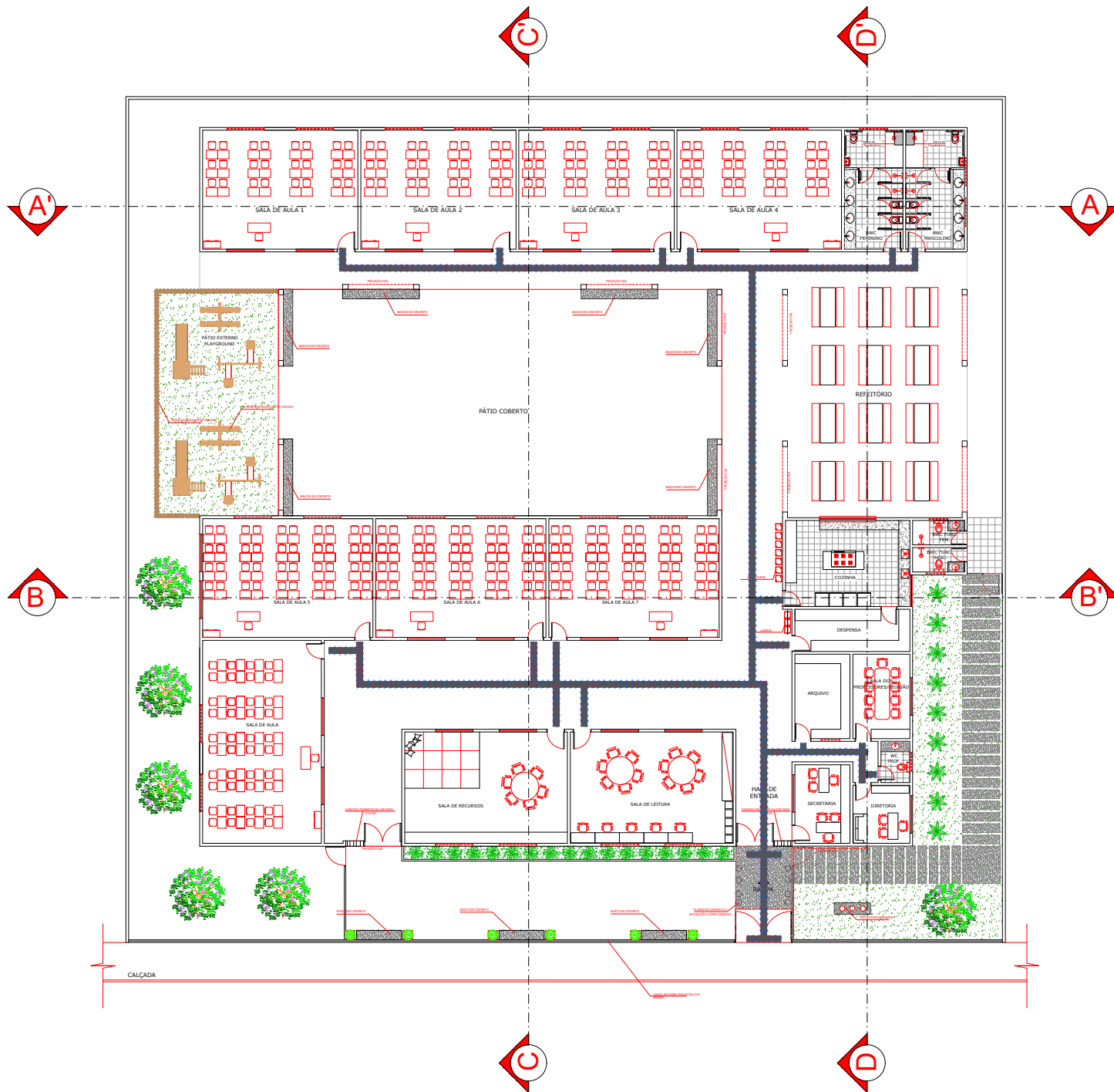
1 PLANTA BAIXA - PISO TÁTIL ESCALA 1/50
