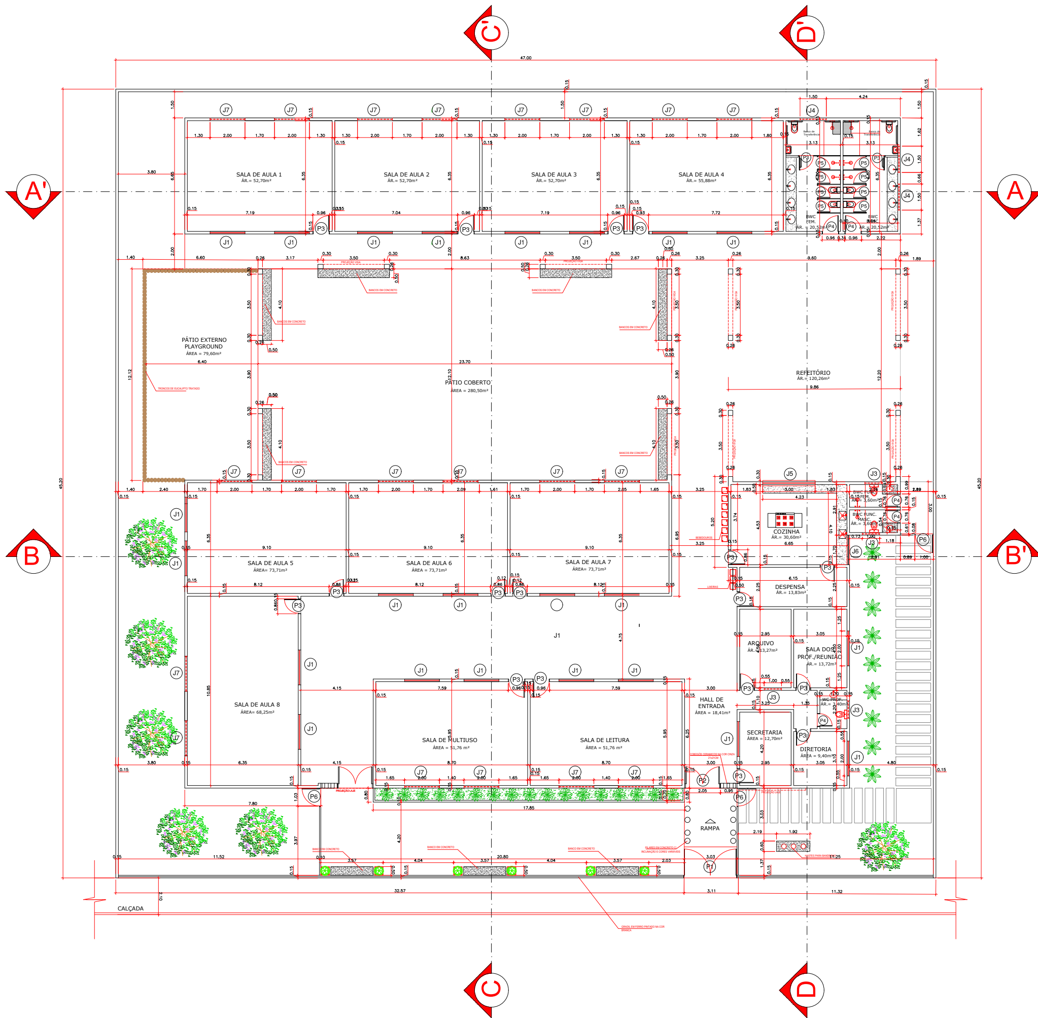
1 PLANTA BAIXA ESCALA 1/50
