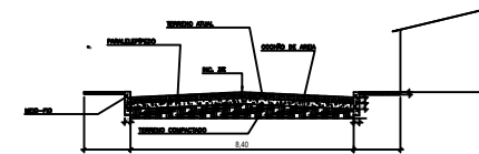
SEÇÃO TRANSVERSAL PADRÃO RUA E (E5 ATÉ E8+17,05)
