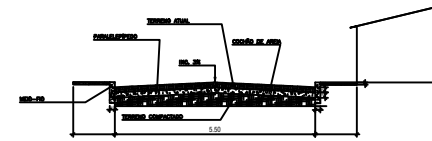
SEÇÃO TRANSVERSAL PADRÃO RUAS C, D, E & F
