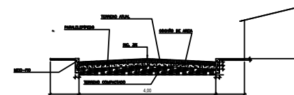
SEÇÃO TRANSVERSAL PADRÃO RUA X
