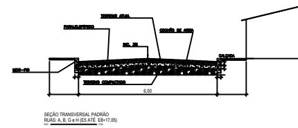
SEÇÃO TRANSVERSAL PADRÃO RUAS A, B, G & H (E5 ATÉ E8+17,05)
