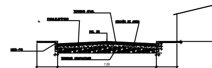
SEÇÃO TRANSVERSAL PADRÃO RUA J
