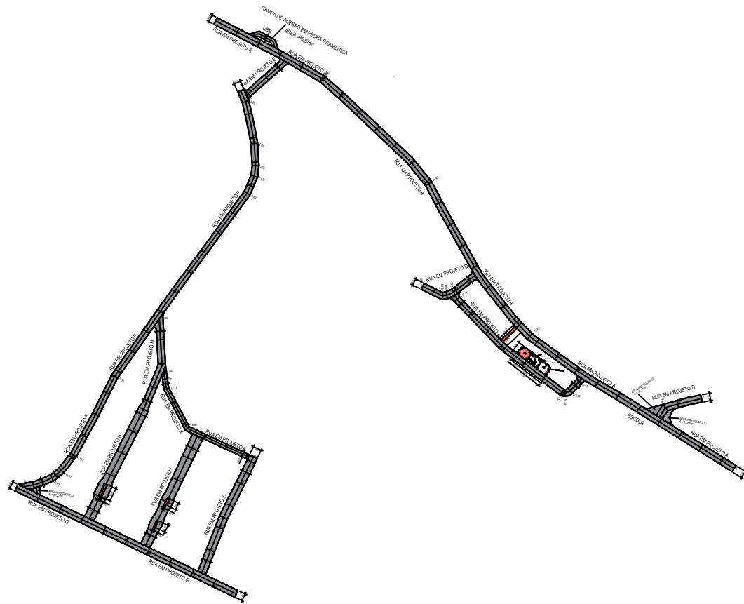
LEVANTAMENTO PLANIMÉTRICO DAS RUAS PROJETADAS A, B, C, D, E, F, G, H, I, J e K NO POVOADO FRUITOSO
